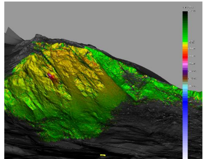
Daten-Visualisierung
